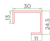
Sash Rein 6002-1502
