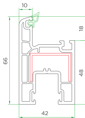
Door sash Rein 6001-1504
