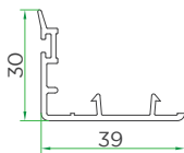
Sash Interlock VVI155-0050
