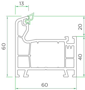
Casement Frame VVI260-2010
