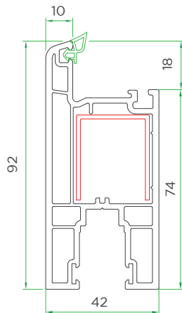
Big door sash Rein 6001-1504
