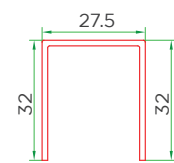
Big door sash Rein 6001-1504
