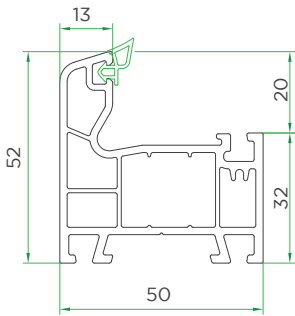
Casement Frame VVI250-2010
